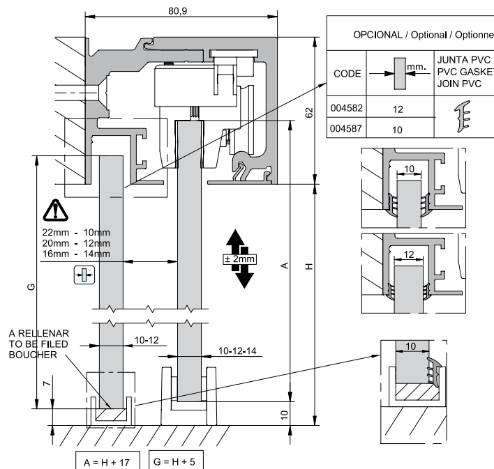
SV - X150 Montaje a pared opción vidrio fijo
