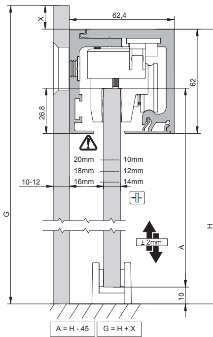
SV - X150 Montaje a pared opción vidrio fijo
